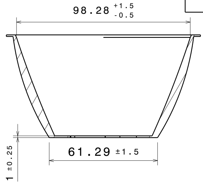
Section view A-A Scale: 3:4
