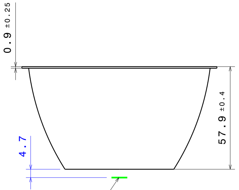
Bottom view Scale: 3:4
